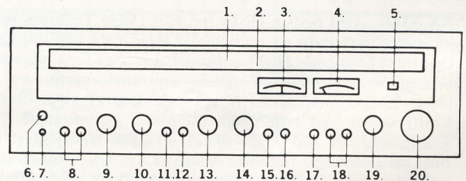
1. Stationskala FM. 2. Stationskala AM. 3. Midtpunktsinstrument. 4. Feltstyrkeinstrument. 5. Kontrollampe for FM stereo. 6. Afbryder. 7. Hovedtelefonbøsning. 8. Højttaleromskifter. 9. Baskontrol. 10. Diskantkontrol. 11. Low filter. 12. High filter. 13. Balancekontrol. 14. Styrkekontrol. 15. Loudness. 16. Muting. 17. Mono/stereoomskifter. 18. Tape Monitor knapper. 19. Programvælger. 20. Skalaknap.
