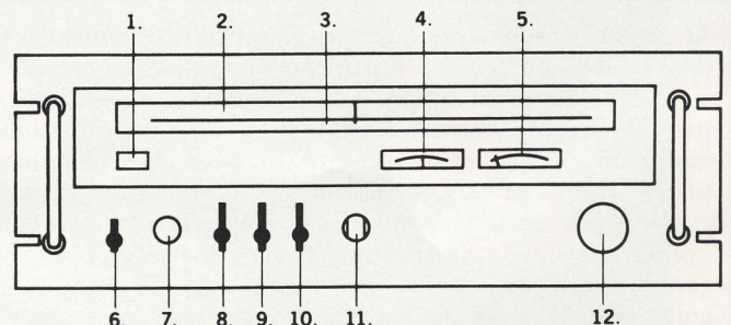
1. Kontrollampe for FM stereo. 2. Stationsskala FM. 3. Stationsskala AM. 4. Midtpunktsinstrument. 5. Feltstyrkeinstrument. 6. Afbryder. 7. Kontrol for udgangsniveau. 8. Omskifter for FM stereo støjfilter. 9. Omskifter for Servo-Tuning og Muting. 10. Omskifter for båndoptager. 11. Programvælger. 12. Skalaknap.
