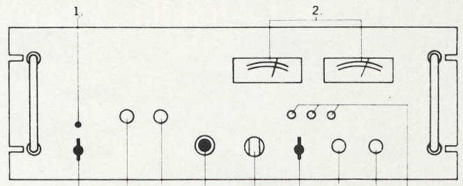
1. Kontrollampe. 2. Spidsværdvisende instrumenter for udgangseffekt. 3. Afbryder. 4. Højttaleromskifter. 5. Hovedtelefonbøsning. 6. Omskifter for udgangsimpedans. 7. Afbryder for det tilførte signal. 8. Niveauekontrol for venstre kanal. 9. Niveauekontrol for højre kanal. 10. Følsomhedsomskiftere for instrumenterne.
